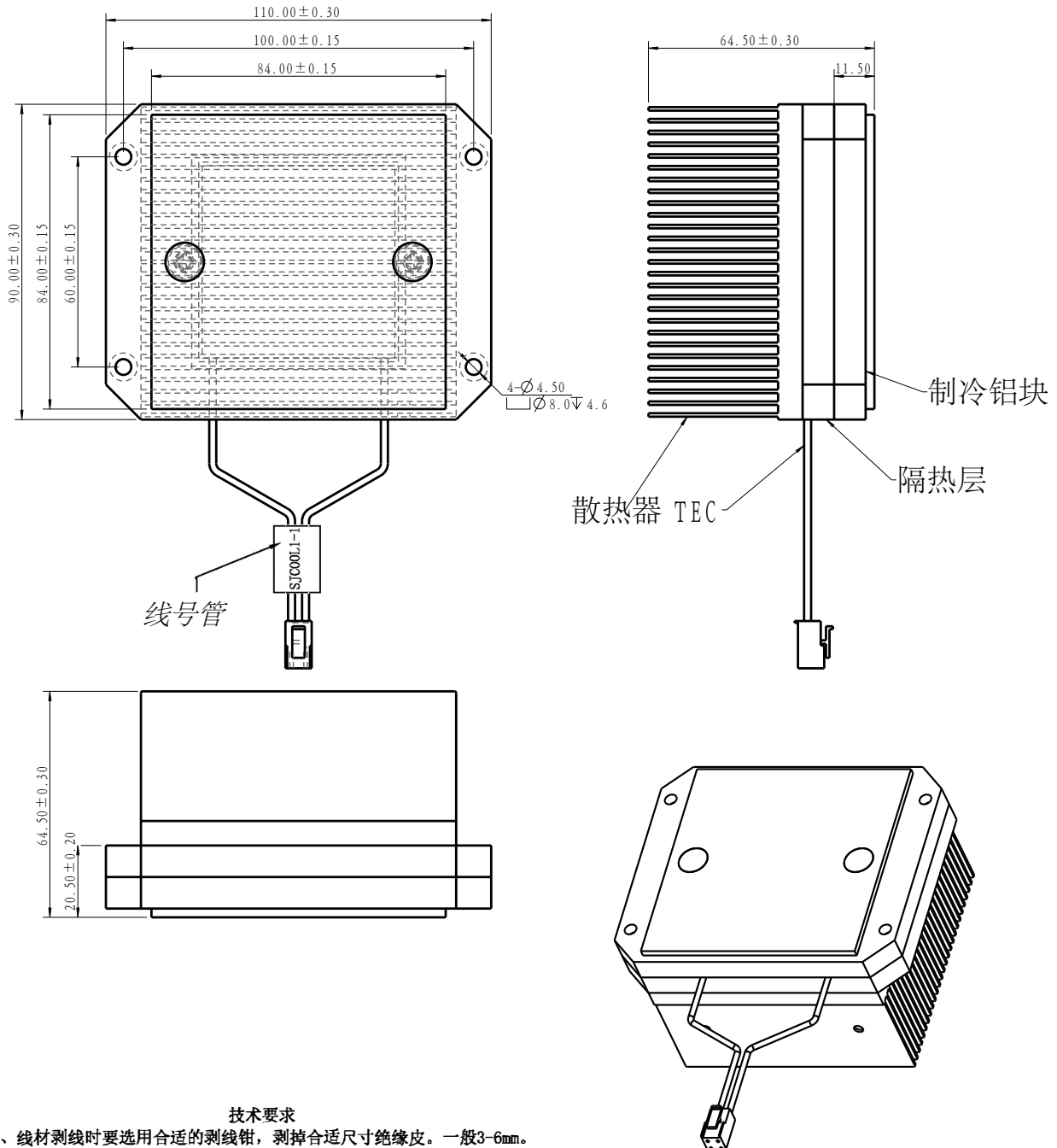
整机外形尺寸图
